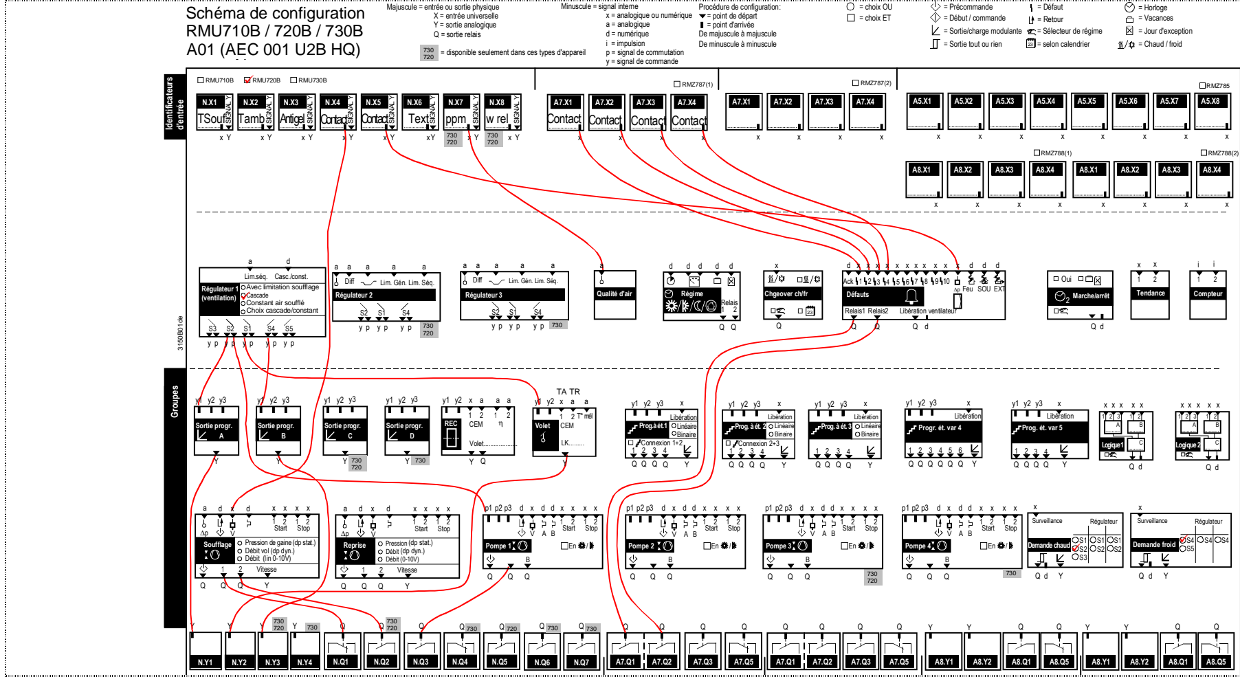
29.2.12 Schéma de configuration RMU720B, type d'installation A01
