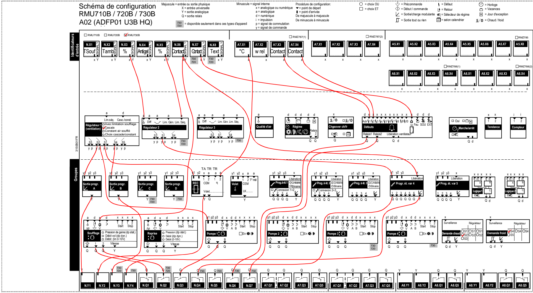
29.2.18 Schéma de configuration RMU730B, type d'installation A02
