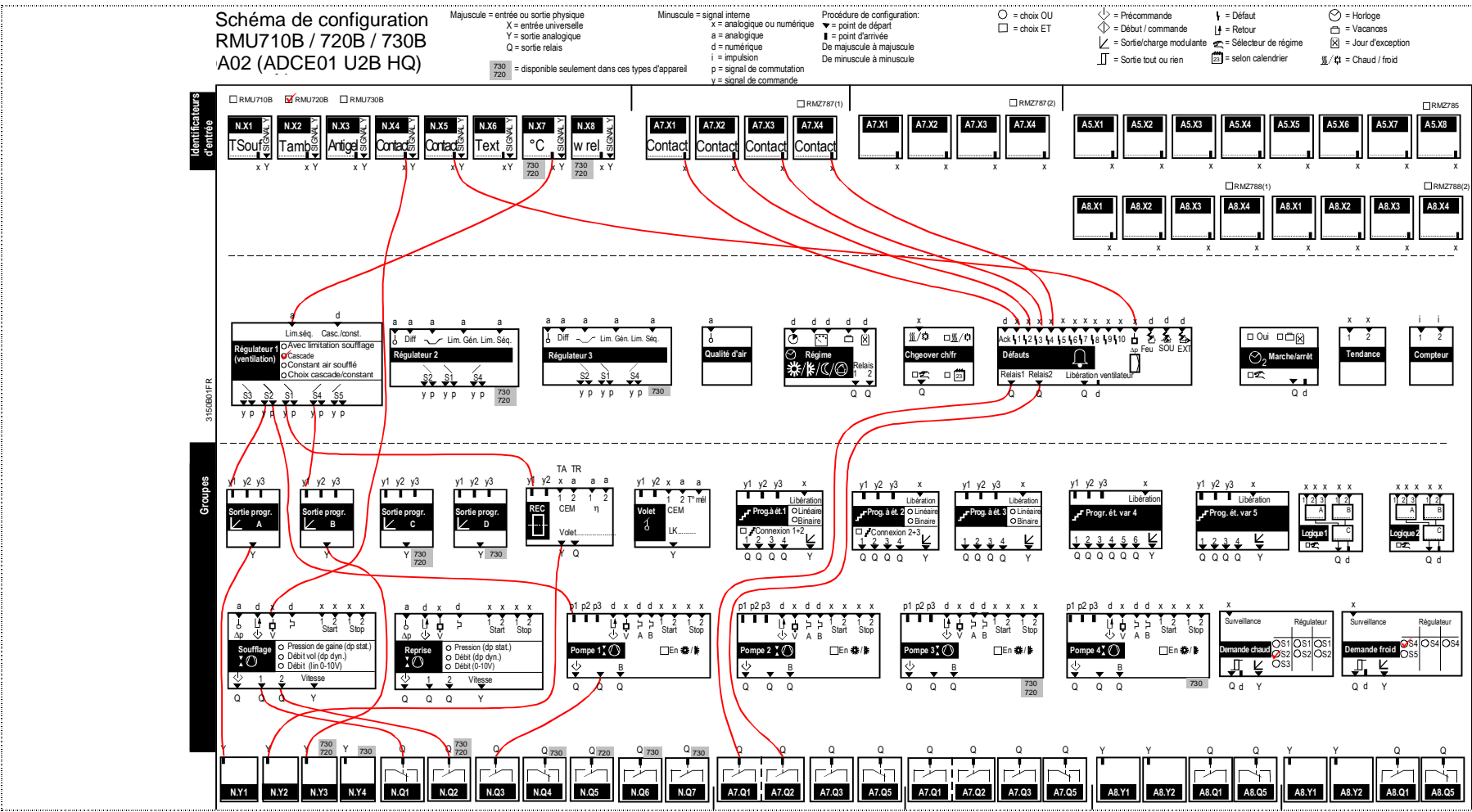
Figure 11 : Schéma de configuration pour la fiche d'application ADCE01 U2B HQ
