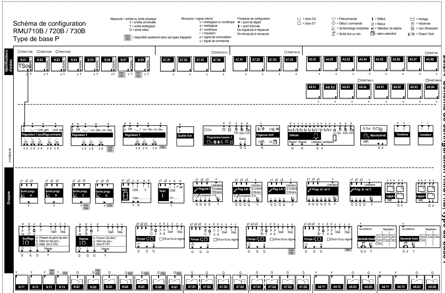
29.2.4 Schéma de configuration RMU7.B, type de base P
