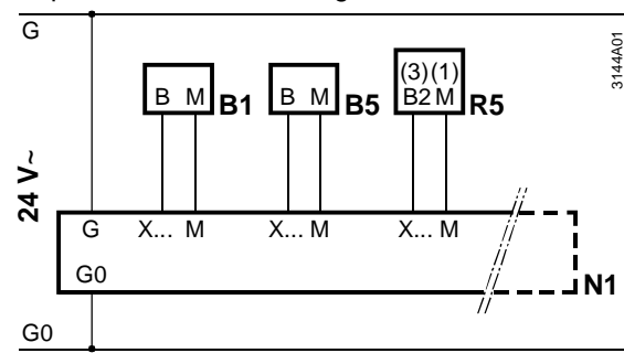
R5 Potentiomètre de consigne passif BSG21.5
