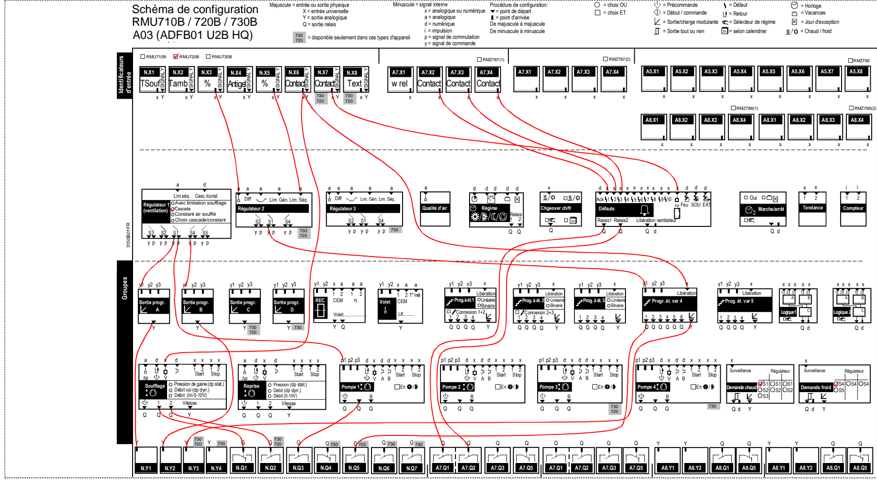
29.2.14 Schéma de configuration RMU720B, type d'installation A03
