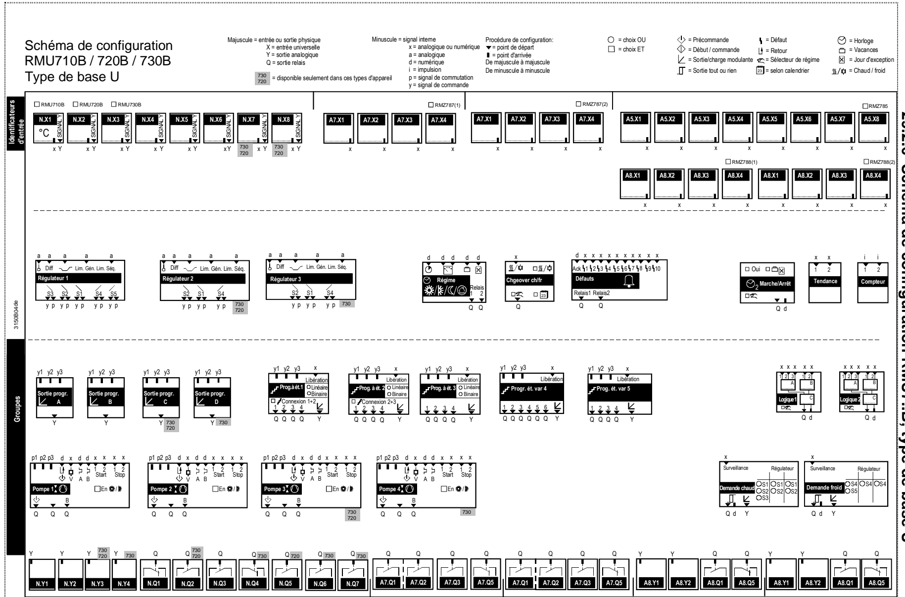
Figure 4: Schéma de configuration du type de base U pour RMU7..B
