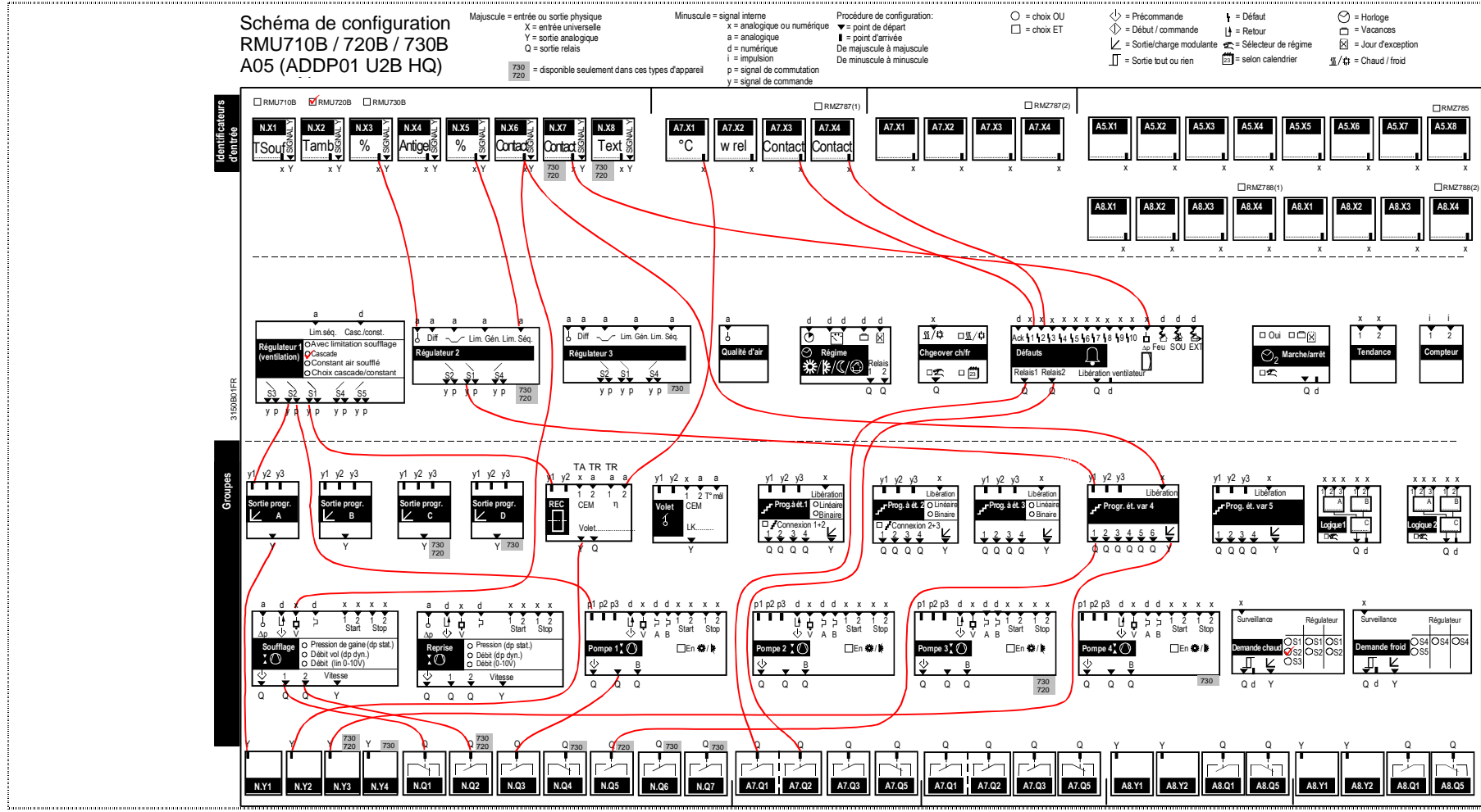
29.2.16 Schéma de configuration RMU720B, type d'installation A05
