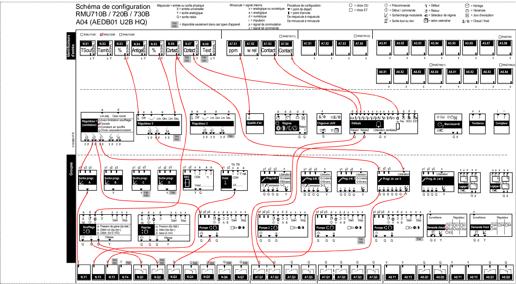
Figure 13: Schéma de configuration pour la fiche d'application AEDB01 U2B HQ
