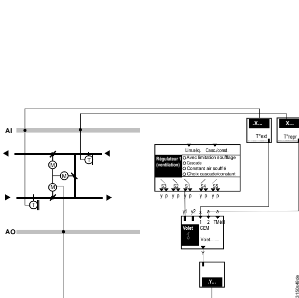
Commande par séquences de chauffage (S1, S2, S3)
