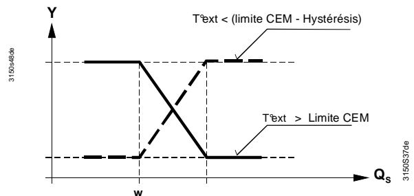
Commande par séquences de refroidissement (S4, S5)
