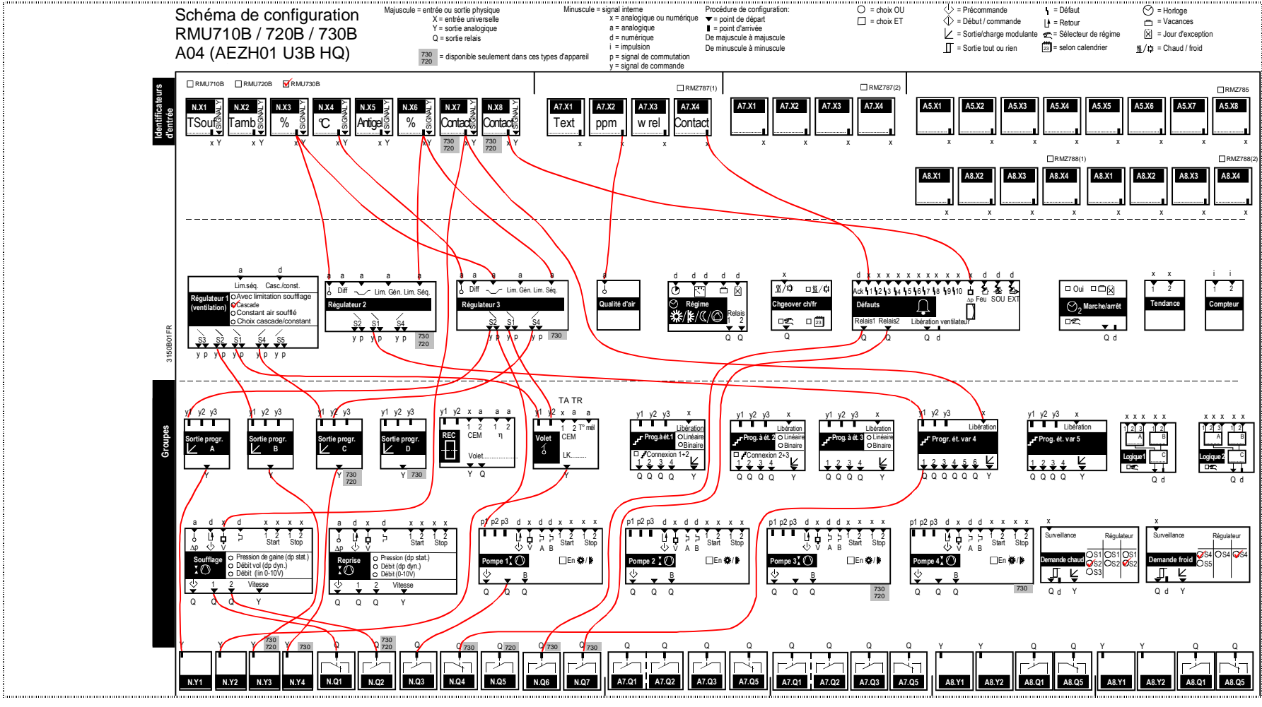
29.2.20 Schéma de configuration RMU730B, type d'installation A04
