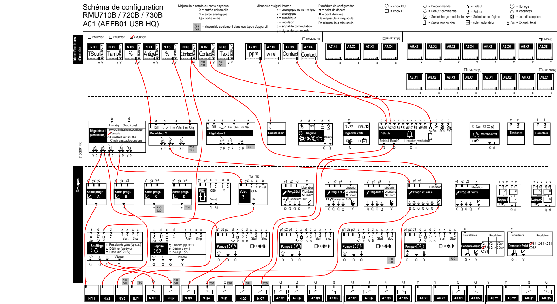
29.2.17 Schéma de configuration RMU730B, type d'installation A01
