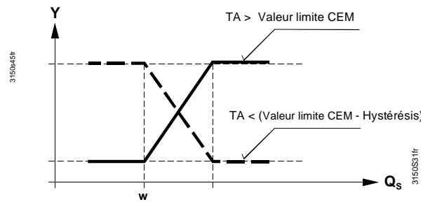
Commande par les séquences de refroidissement (S4, S5)
