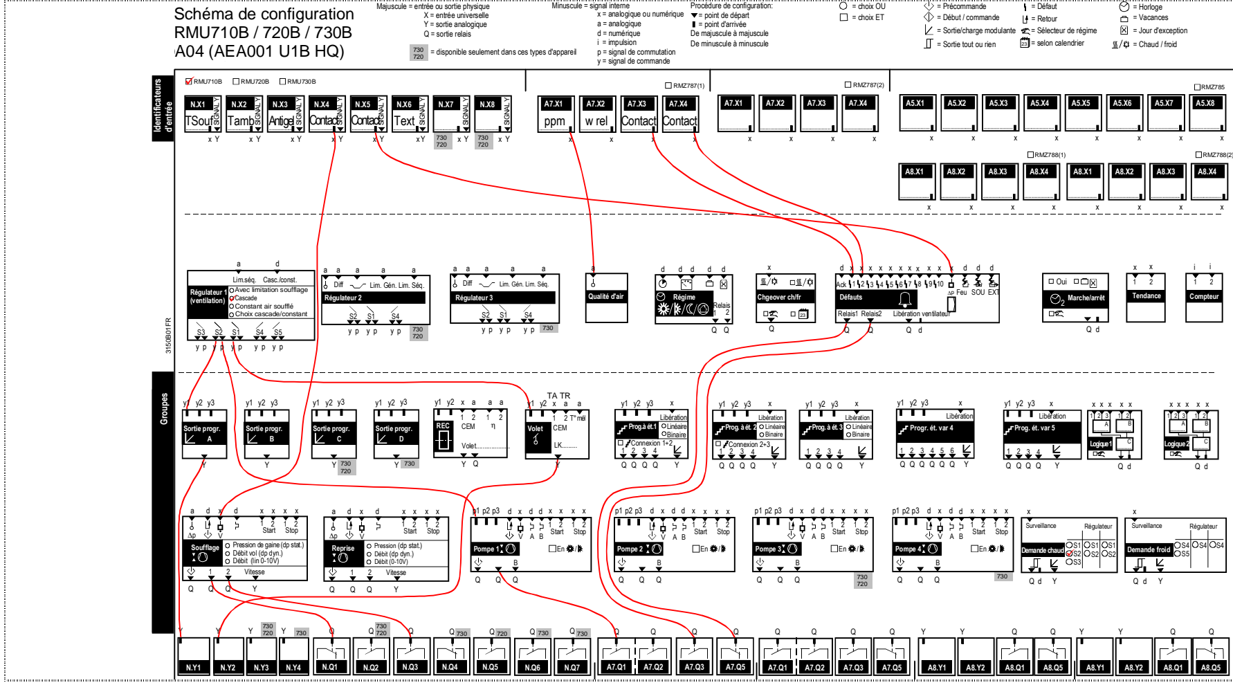
29.2.10 Schéma de configuration RMU710B, type d'installation A04
