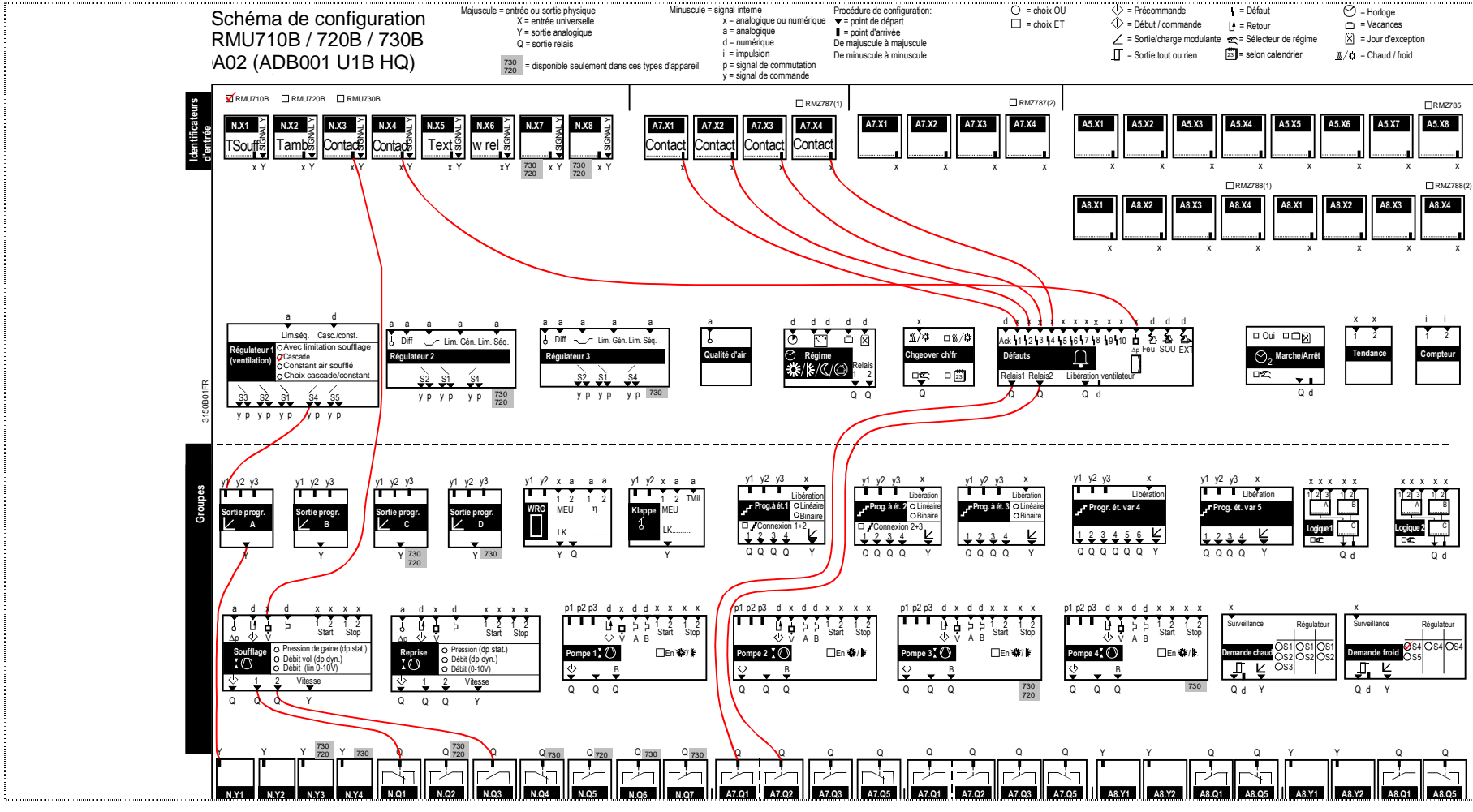
29.2.8 Schéma de configuration RMU710B, type d'installation A02
