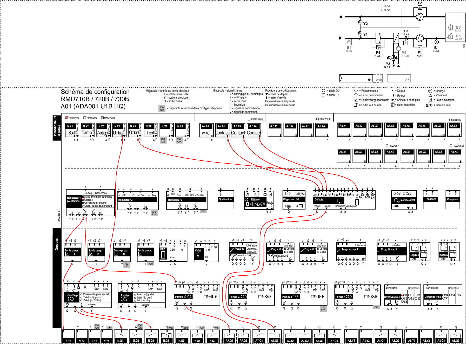
Figure 5: Schéma de configuration pour la fiche d'application ADA001 U1B HQ
